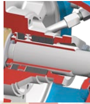
S3 Zachte pakkingringen, asbus, lantaarn ring
