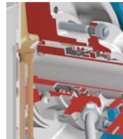
MQ2 MG12 / M7N Enkele mechanische asafdichting, ongebalanceerd, droogloopbeveiliging, asbus
