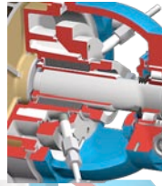
S4 Zachte pakkingringen, asbus, koelmantel
