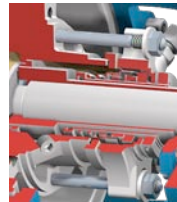
Cartridge asafdichtingen Enkel, enkel met vloeistofspoeling en dubbel cartridge asafdichtingen
