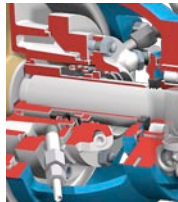
MW2 MG12 / M7N Enkele mechanische asafdichting, ongebalanceerd, koelmantel, asbus
