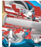
MW3 HJ92N / HJ977GN Enkele mechanische asafdichting, gebalanceerd, koelmantel, asbus
