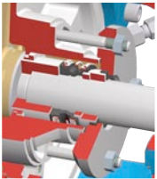
M1 Enkele mechanische asafdichting, ongebalanceerd
