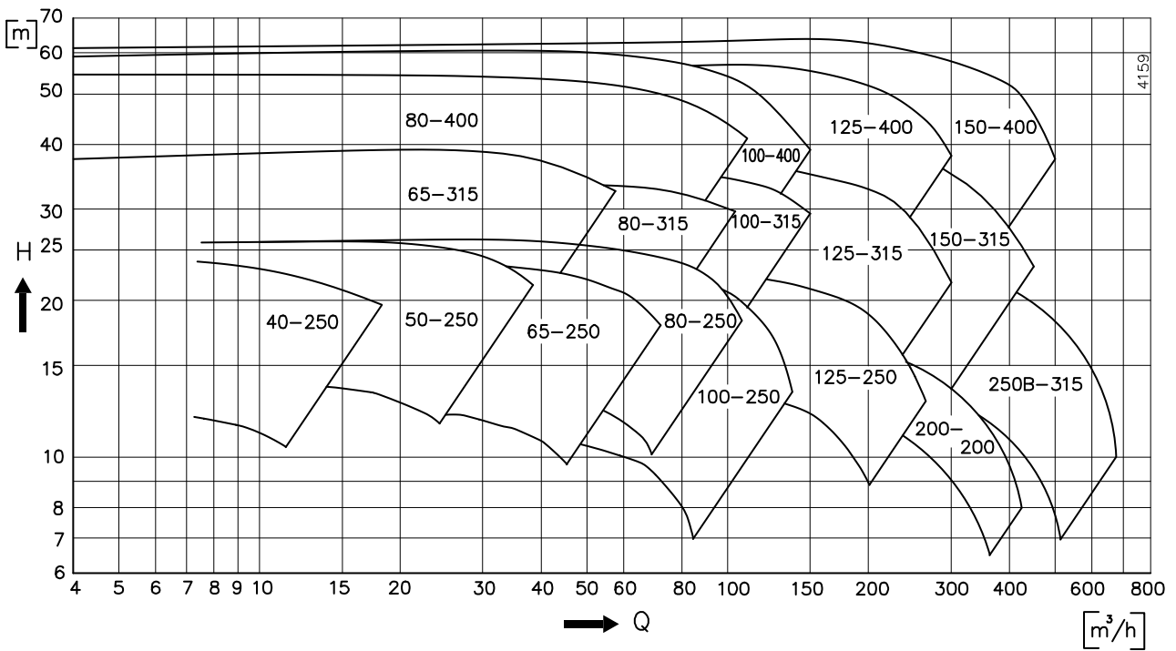
Figuur 36: Overzichtsgrafiek 3000 min -1 .
