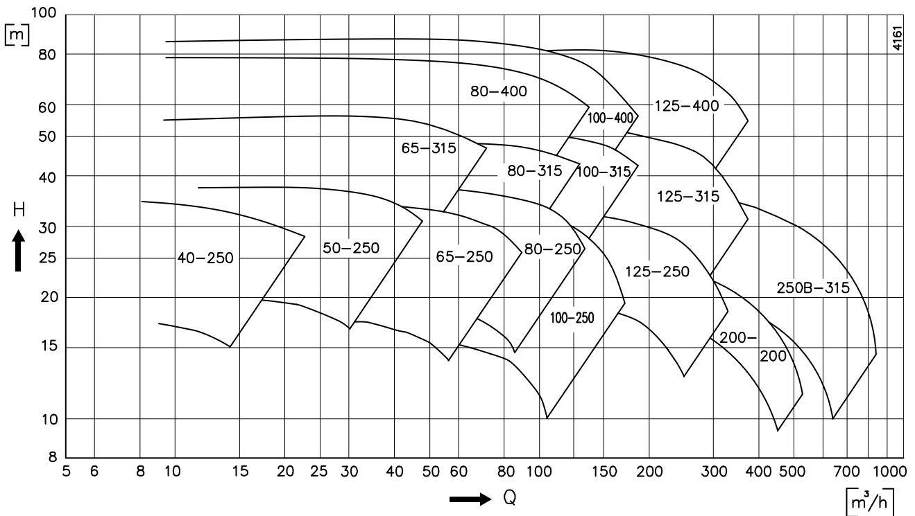
Figuur 38: Overzichtsgrafiek 3600 min -1 .
