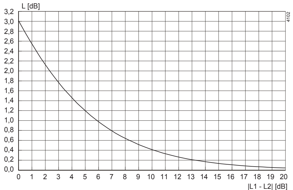
Figuur 42: Geluidsniveau van de totale pompunit.
