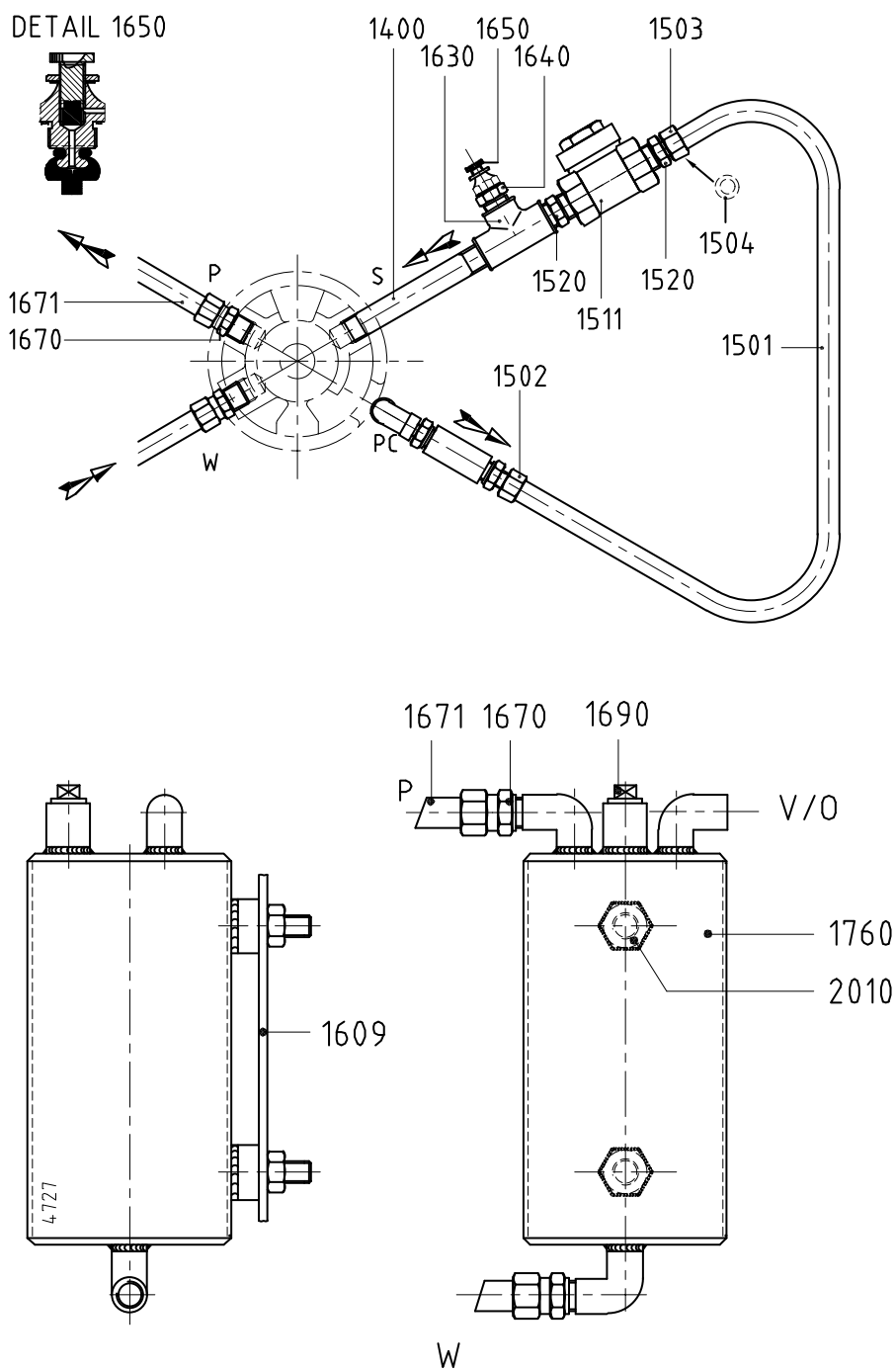
Figuur 32: Bedrijfsvloeiستoftank TL.
