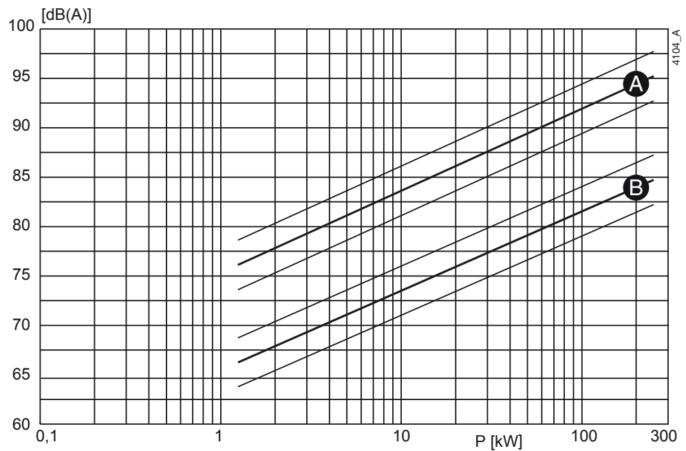
Figuur 41: Geluid als functie van het pompvermogen bij 2900 \text{ min}^{-1} A = geluidsvermogen, B = geluidsdruk.
