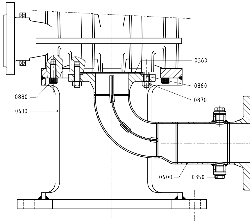
Figuur 35: Doorsnedetekening zuigbocht 200-200 / 250B-315.
