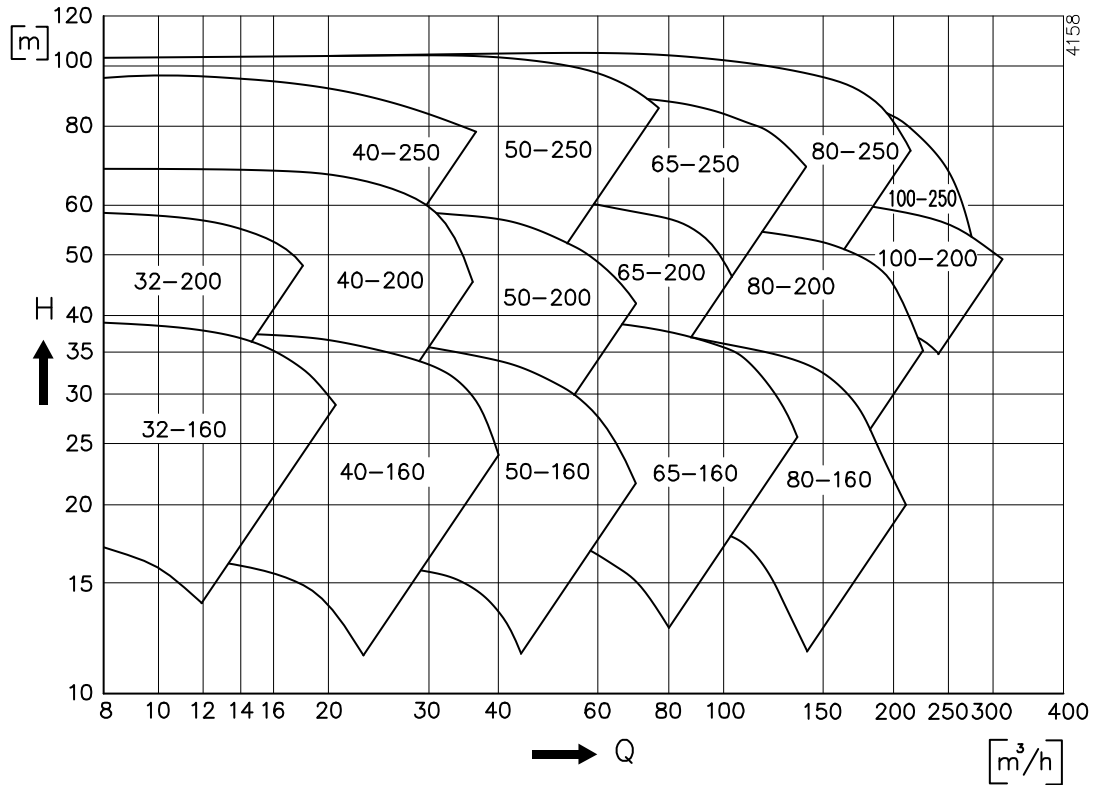
Figuur 36: Overzichtsgrafiek 3000 min -1 .
