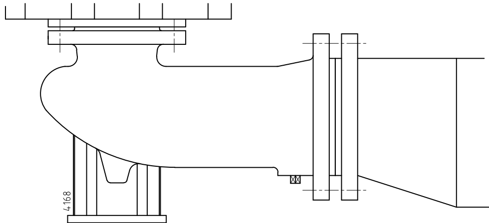
Figuur 3: Excentrisch verloopstuk naar de zuigflens.
