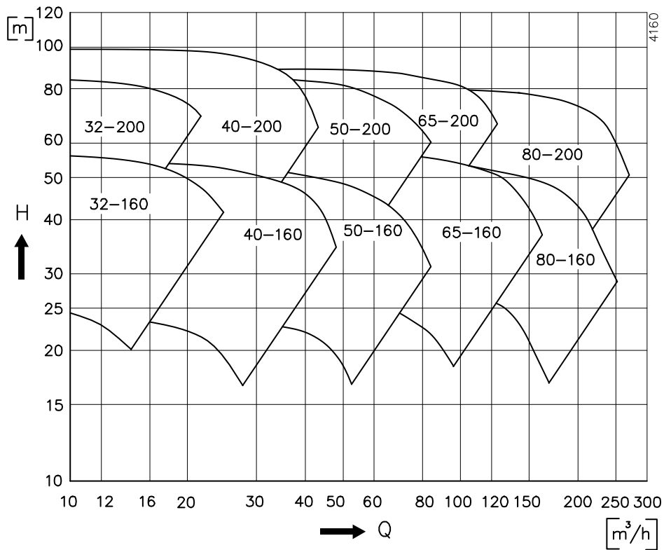
Figuur 38: Overzichtsgrafiek 3600 min -1 .
