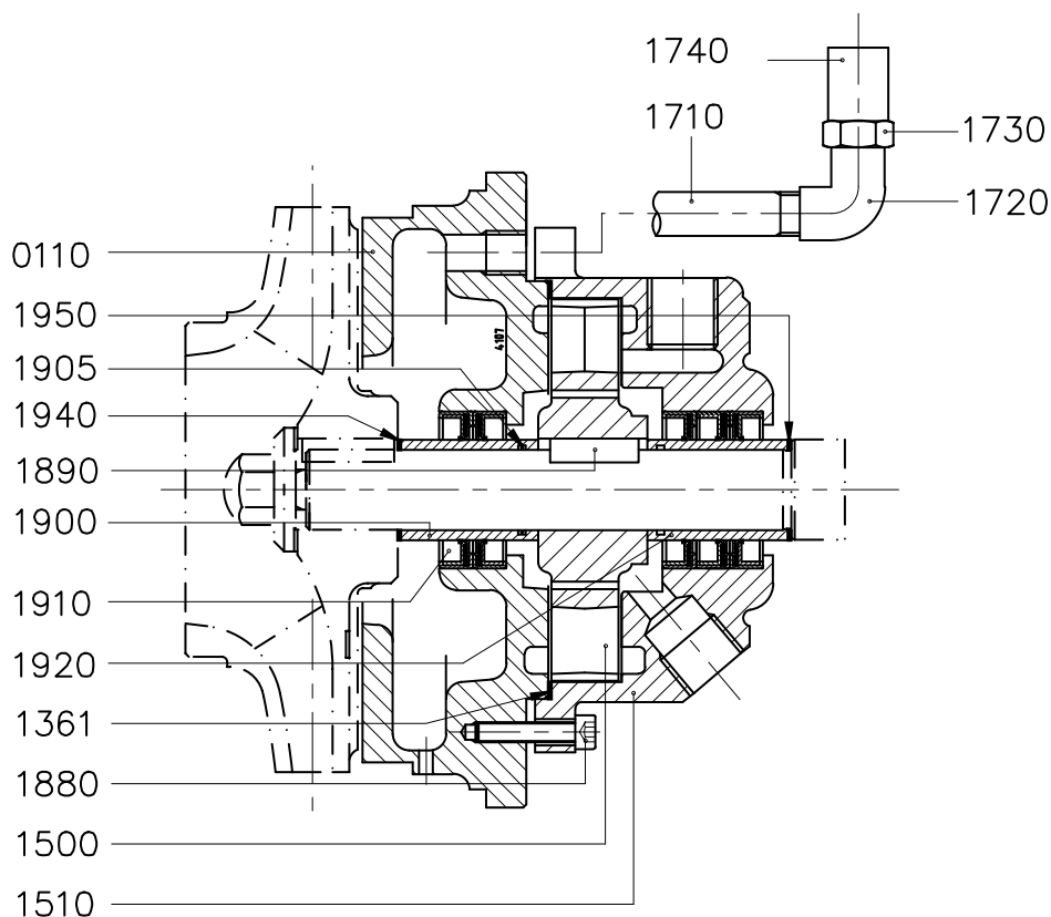
Figuur 17: Lipringafdichting M4.
