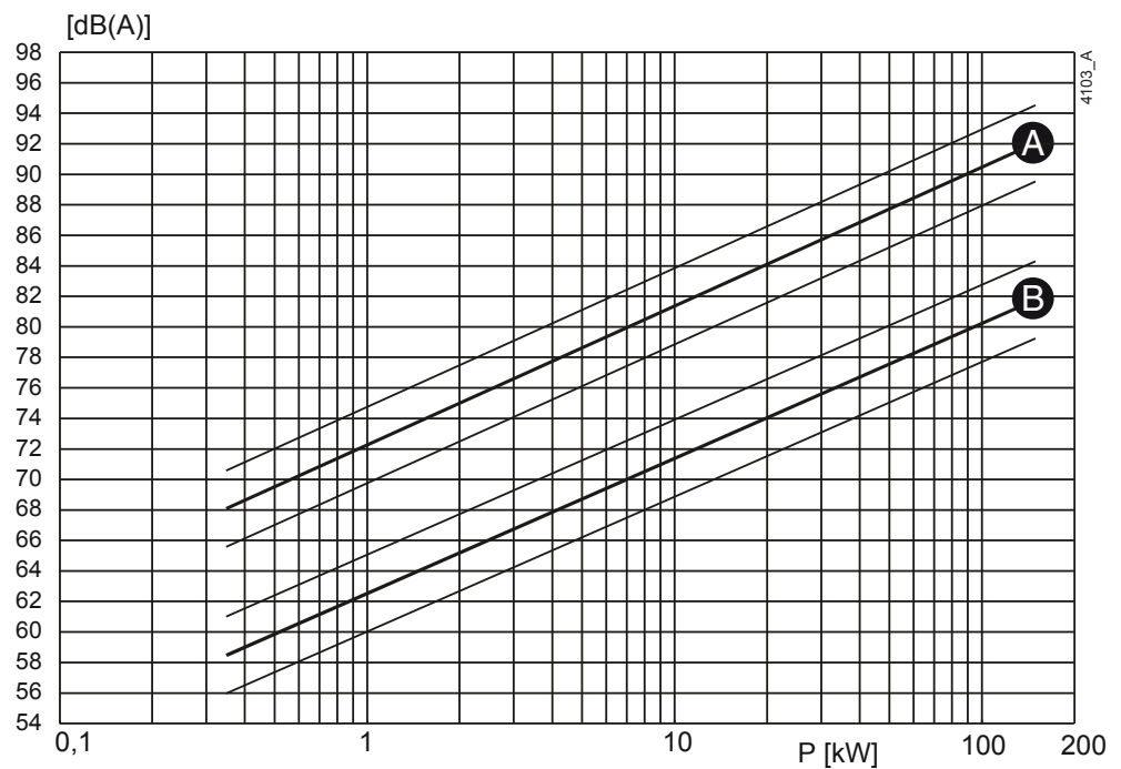
Figuur 40: Geluid als functie van het pompvermogen bij 1450 \text{ min}^{-1} A = geluidsvermogen, B = geluidsdruk.
