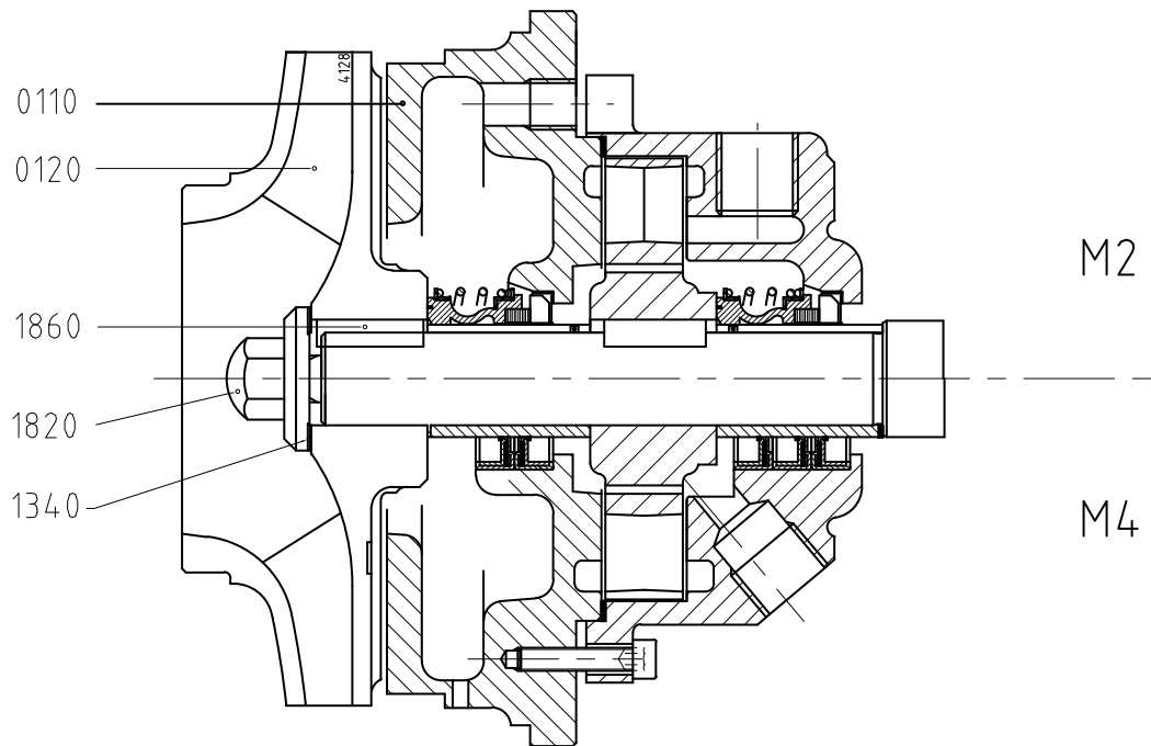
Figuur 14: Demontage van de waaier.
